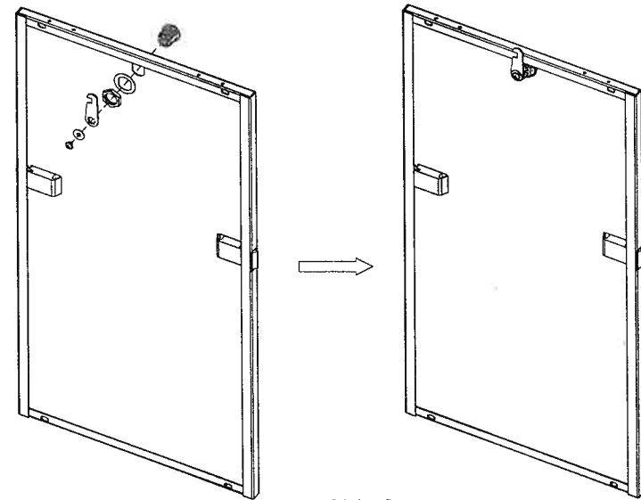
Side Door
